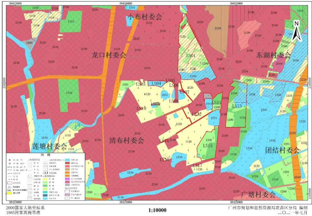
广州市花都区花山镇、新雅街道落实地块土地利用规划图（局部一，落实前）
