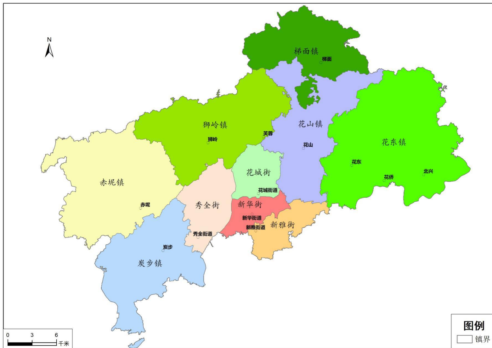
图 1 花都区行政区划图
