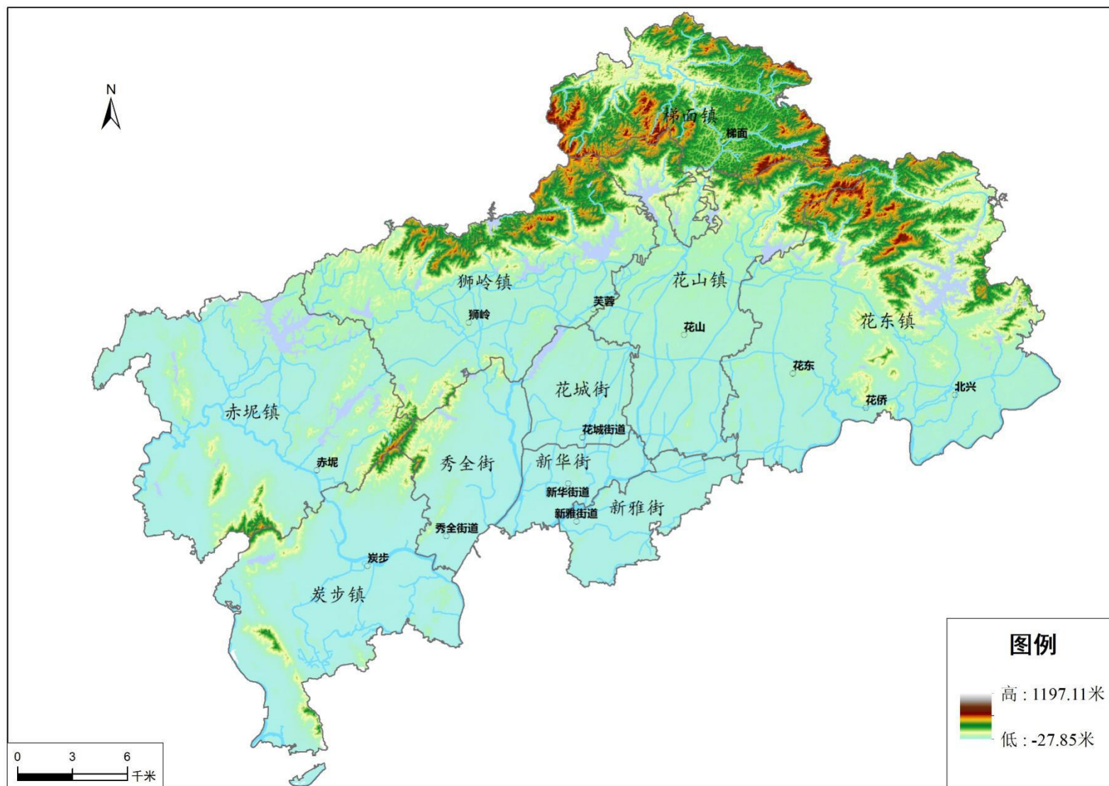
图 3 花都区数字高程图
